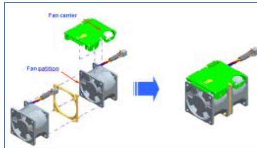
Figure 23. Fan Module for R510-12
